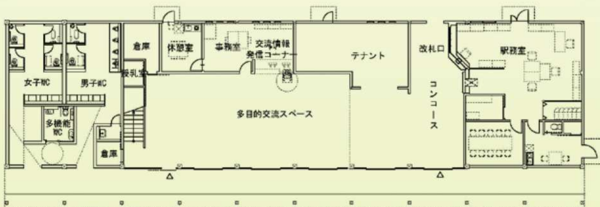
1階平面図
