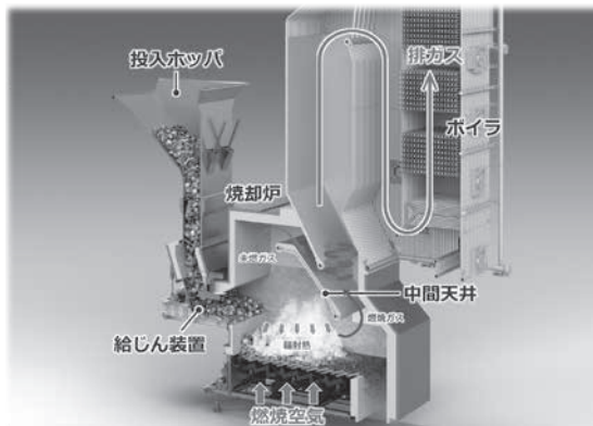
ストーカ式焼却炉の構造
