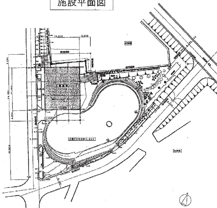
施設平面図
