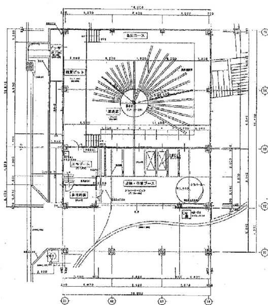
建物平面図
